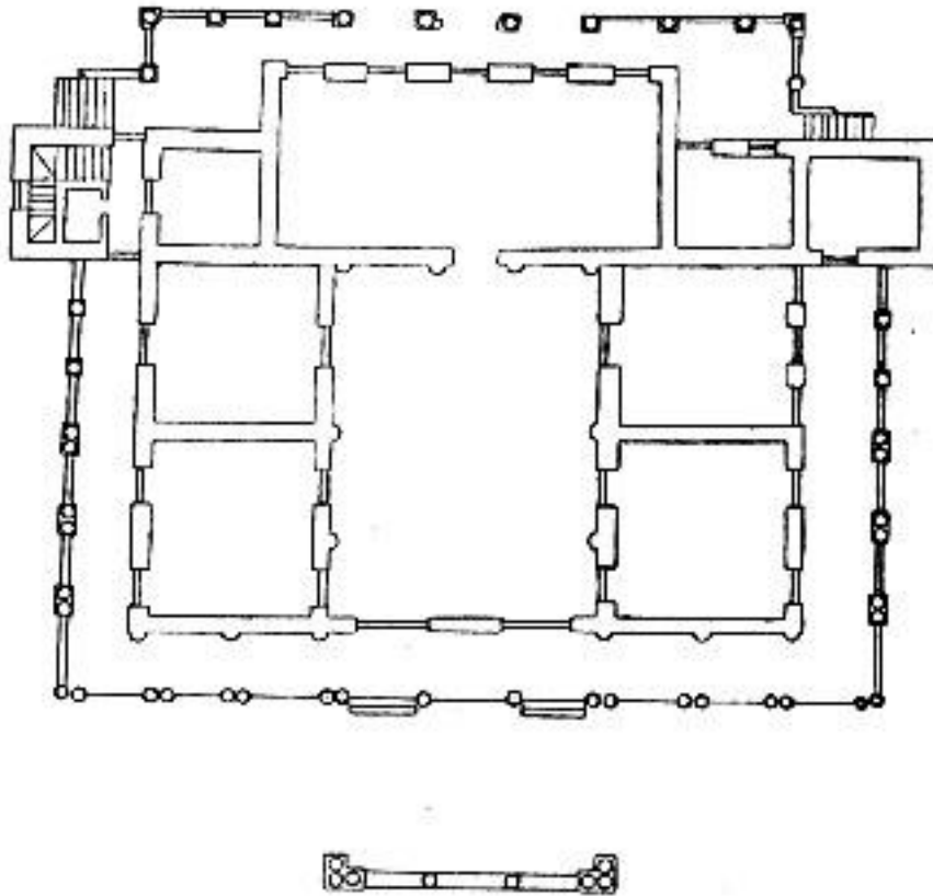
ПЛАН НУЛЕВОГО ЭТАЖА ЗДАНИЯ ШТАБ-КВАРИТИРЫ, 1882 Г.
